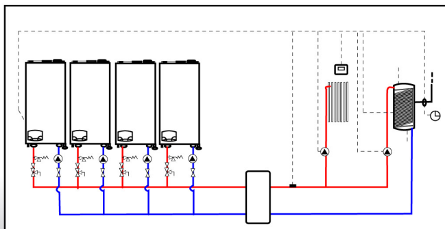
Esquema con 2 bombas en secundario.
