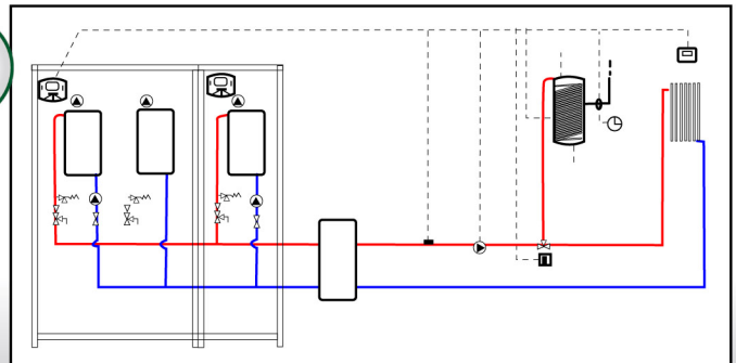
Esquema con bomba y válvula de 3 vías en secundario.
